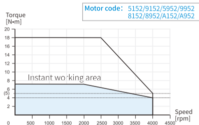
MS6G-130CM/CN/TL/TH20B(Z)2-41P5
