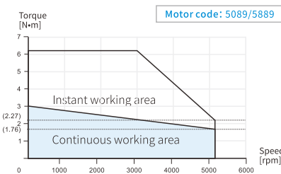
MS6H-80CM30B(Z)4-20P7
