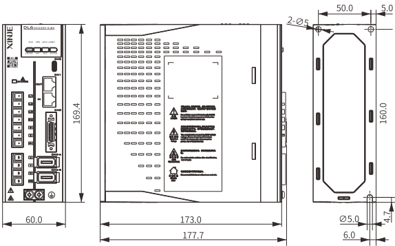
DL6-2003/2006
