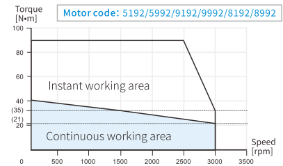
MS6H-180CN/CM15B/E(Z)2-45P5 MS6H-180TL15B(Z)2-45P5
