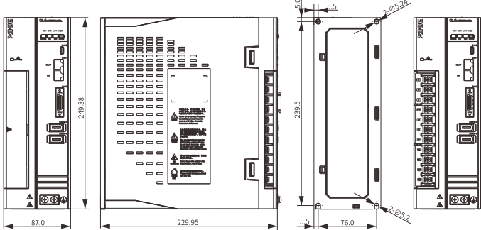
DL6-4020
