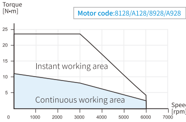
MS6L-100CN/TH30B(Z)2-42P5
