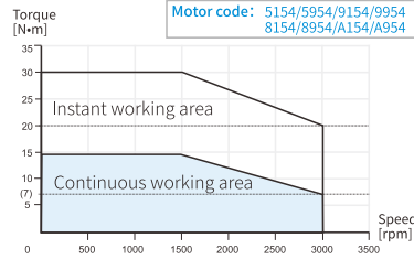
MS6G-130CM/CN/TL/TH15B(Z)2-42P3
