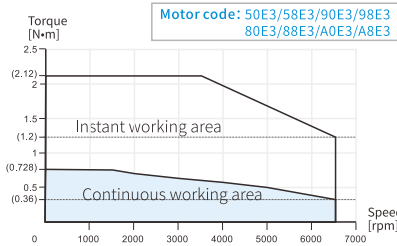
MS6H-60CM/CN/TH/TL30B(Z)3-20P2
