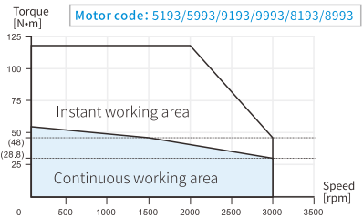
MS6H-180CN/CM15B/E(Z)2-47P5 MS6H-180TL15B/E(Z)2-47P5
