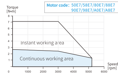
MS6H-80CM/CN/TH/TL30B(Z)3-20P7
