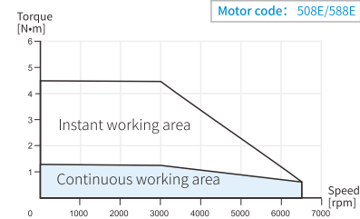
MS6S-60CM30B(Z)4-20P4
