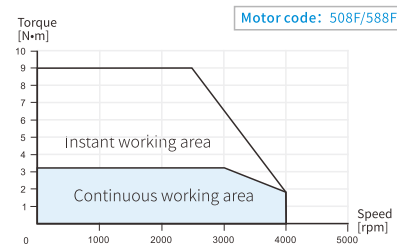
MS6H-80CM30B(Z)4-21P0
