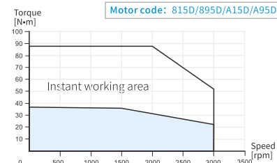
MS6G-180CN/TH15B(Z)2-45P5
