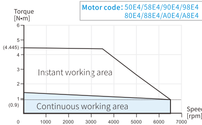
MS6H-60CM/CN/TH/TL30B(Z)3-20P4
