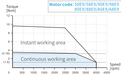
MS6H-80CM/CN/TH/TL30B(Z)3-21P0
